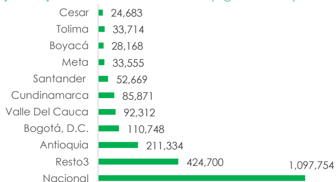
Gráfico 2. Despachos de cemento gris por departamento en toneladas (agosto-2021)
