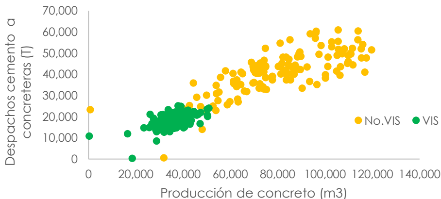
Gráfico 4. Producción de concreto premezclado (m 3 ), serie hasta agosto Vs Despachos de cemento (T) serie hasta julio- Bogotá (Rezago de un mes entre el despacho y la producción 2011 a 2021)
