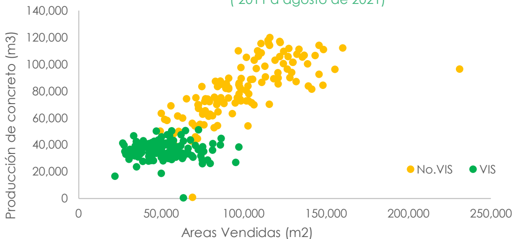
Gráfico 5. Producción de concreto premezclado (m³) Vs áreas vendidas (m²) – Bogotá (2011 a agosto de 2021)
