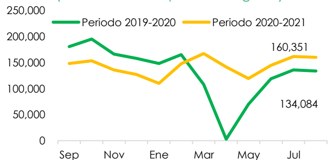
Gráfico 3. Producción mensual de concreto premezclado en metros cúbicos por periodos de doce meses - Bogotá (doce meses – septiembre-agosto)
