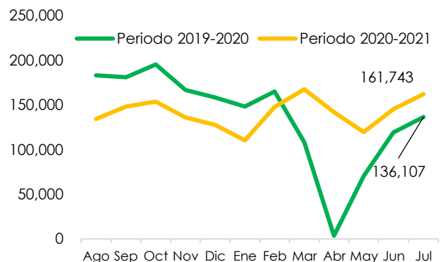
Gráfico 3. Producción mensual de concreto premezclado en metros cúbicos por periodos de doce meses - Bogotá (doce meses – agosto-julio)
