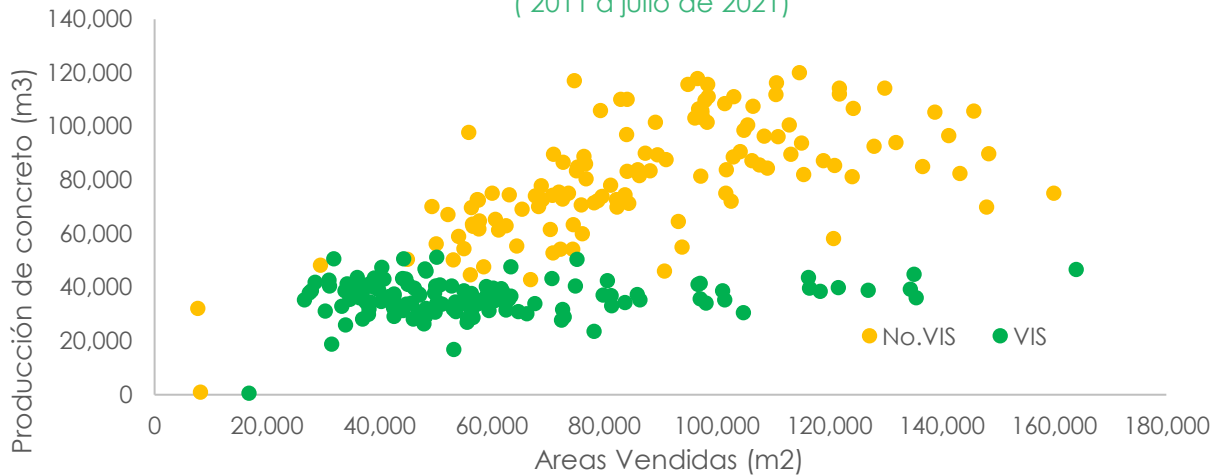
Gráfico 5. Producción de concreto premezclado (m 3 ) Vs áreas vendidas (m 2 )– Bogotá ( 2011 a julio de 2021)
