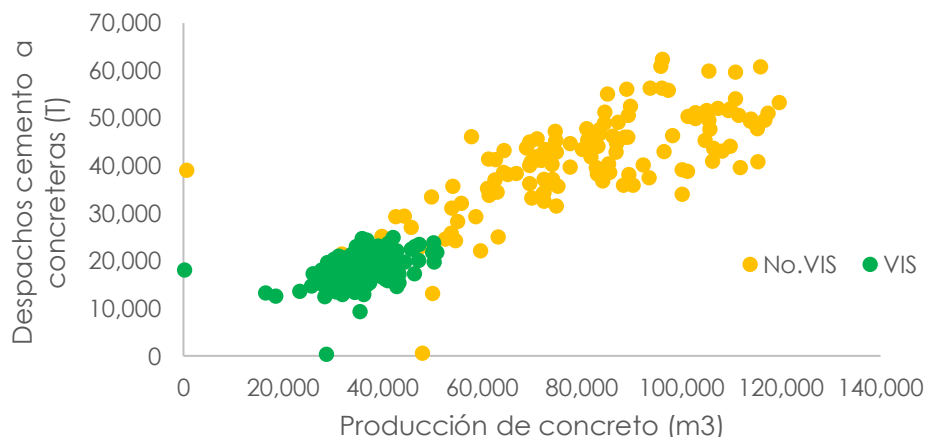
Gráfico 4. Producción de concreto premezclado (m 3 ) en julio Vs Despachos de cemento (T) mayo - Bogotá
