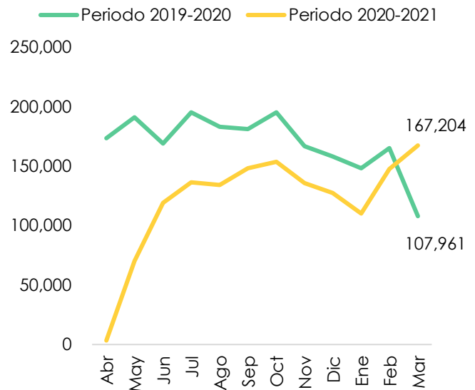
Gráfico 3. Producción mensual de concreto premezclado en metros cúbicos por periodos de doce meses - Bogotá (abril – marzo; 2019-2020- 2021)
