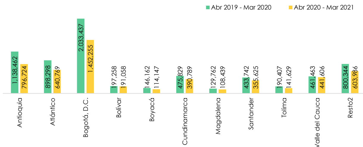
Gráfico 5. Producción de concreto premezclado en metros cúbicos por departamento (doce meses, abril a marzo)
