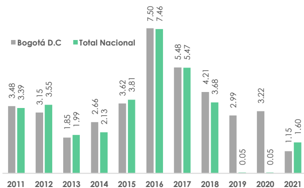
Gráfico 1. Bogotá y total nacional: IPC variación anual enero (2011 – 2021)
