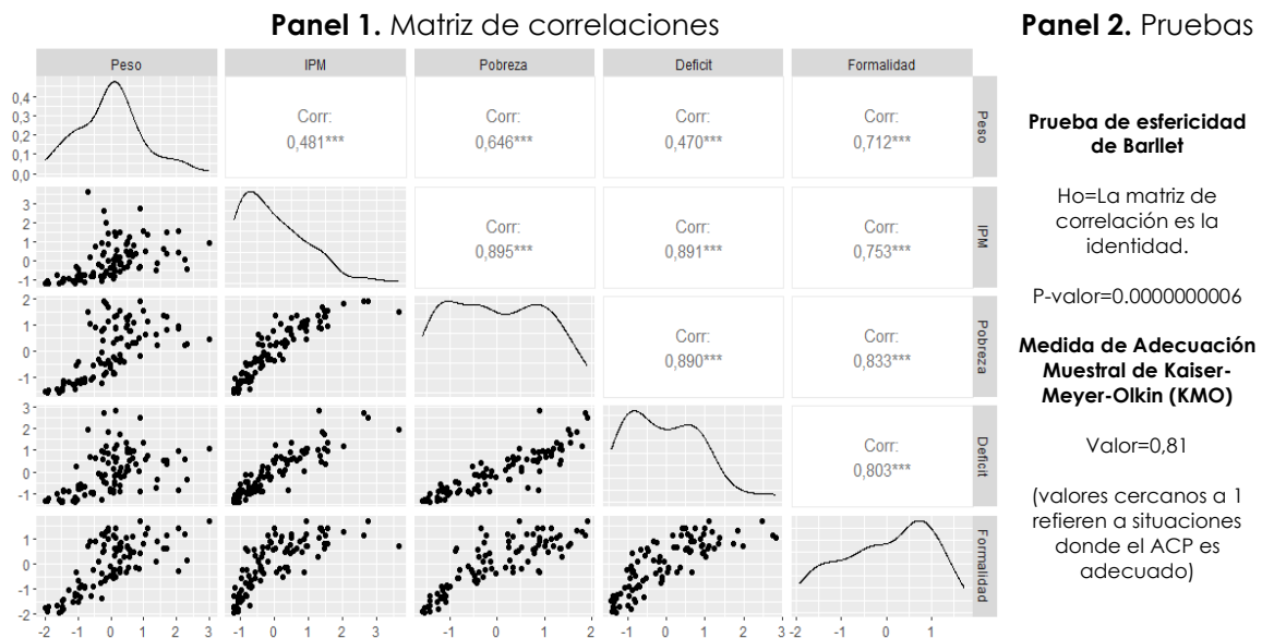
Ilustración 5 Evaluación de la pertinencia del ACP sobre el conjunto de datos
